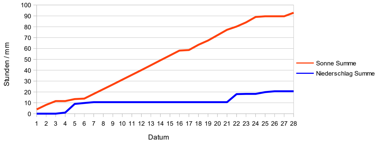
Sonnenschein / Niederschlag Summe Keine Sonnenzeit Daten
